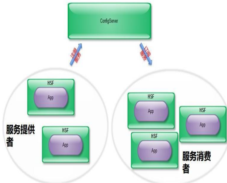
去中心化服务框架
